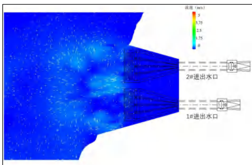
图 5.6-1 发电工况进/出水口附近水平截面流速场
