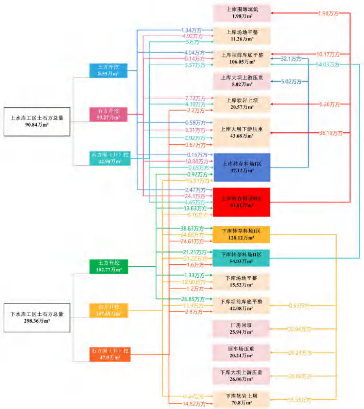
图 2.8-1 土石方调运简图
