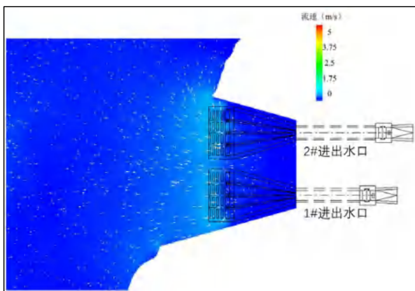
图 5.6-2 抽水工况进/出水口附近水平截面流速场
