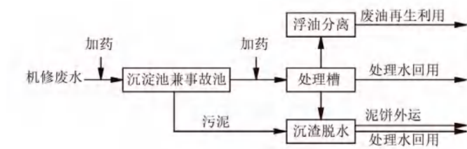
图 6.2-8 机修含油污水处理工艺流程图
