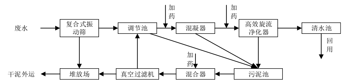
图 6.2-3 高效旋流净化法工艺流程
