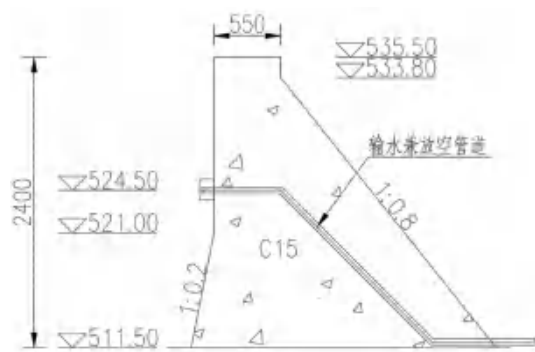
楠木沟非溢流坝段示意图
