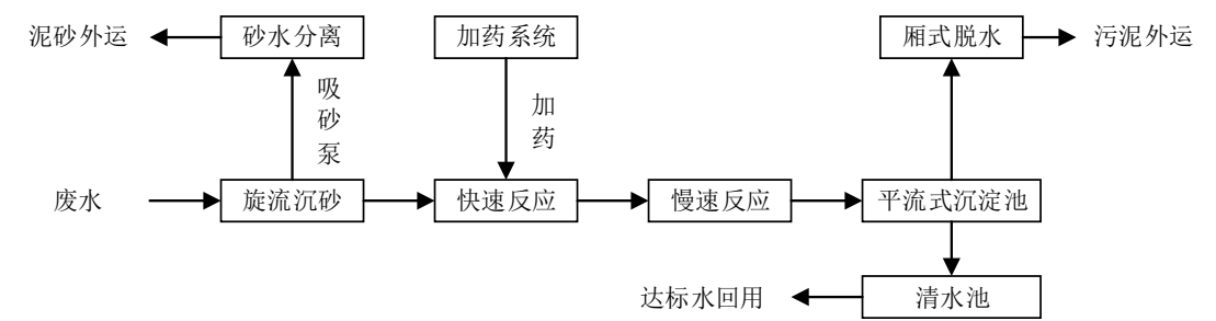
图 6.2-2 絮凝沉淀法工艺流程
