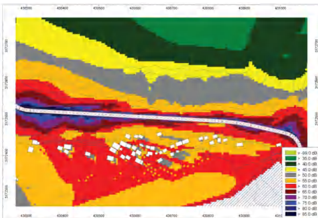
图 5.9-3 进厂公路周边噪声预测等声线图
