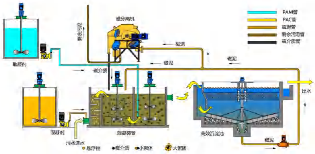
图 6.2-6 砂石加工系统生产废水处理工艺流程图
