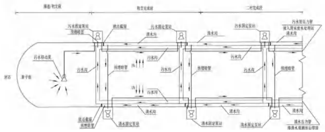
图 6.2-11 钻爆法反坡段清污分流平面示意图
