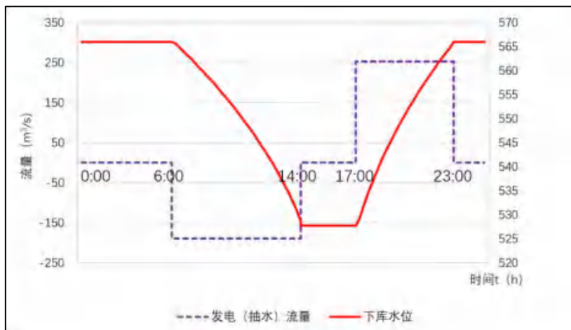
下库水位调度图
