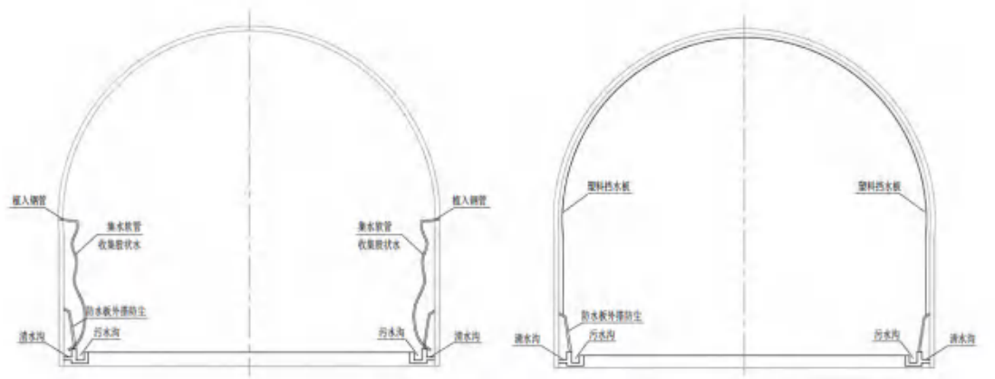
图 6.2-10 钻爆法顺坡初支段清污分流横断面图
