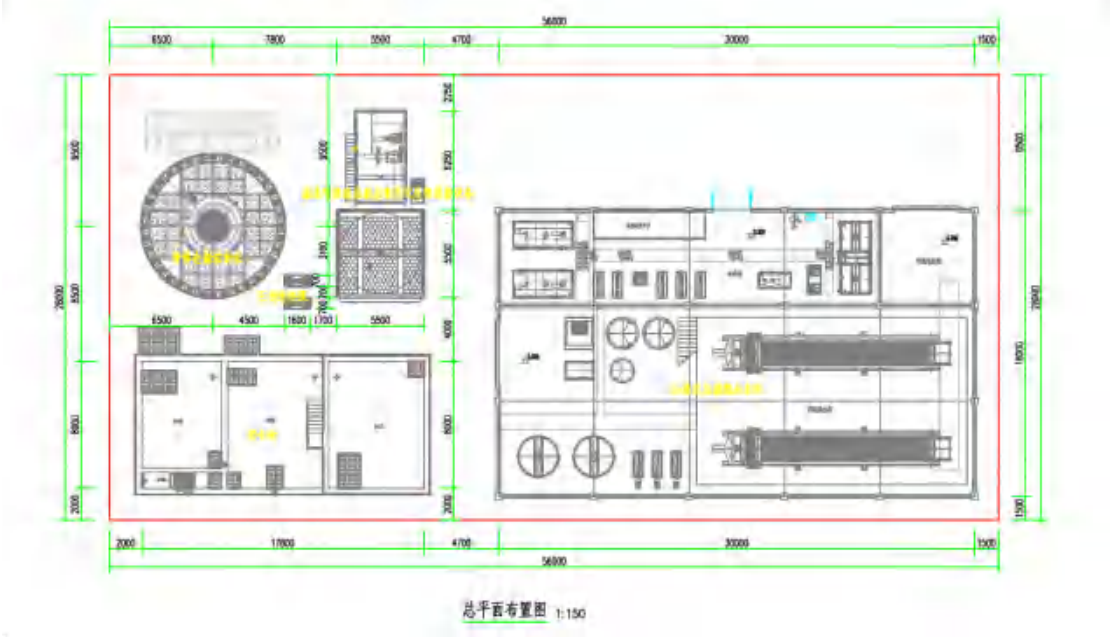
图 6.2-7 砂石加工系统废水处理系统平面布置图
