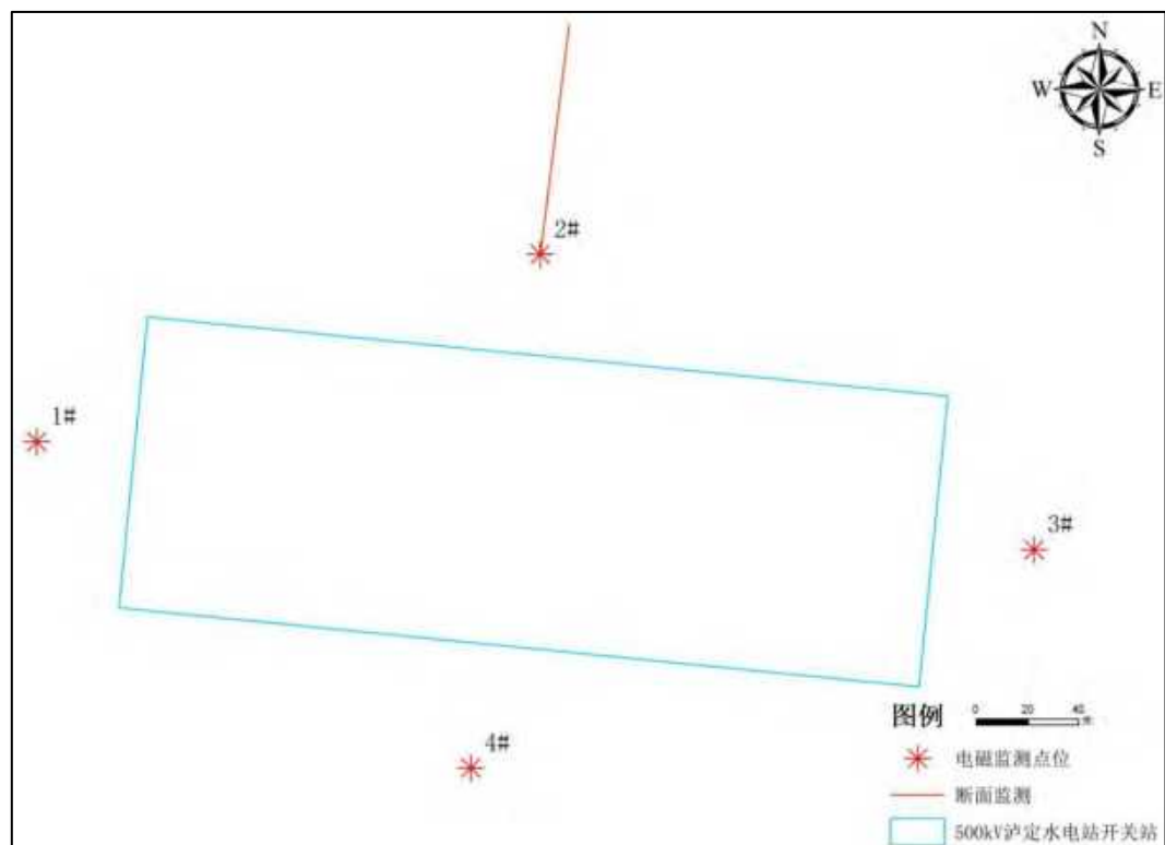
图 5.11-1 类比变电站监测布点图
