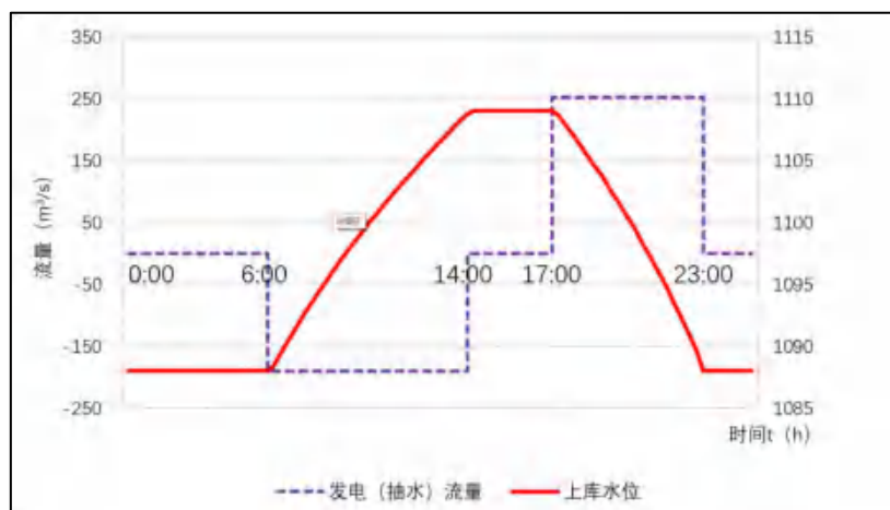
上库水位调度图
