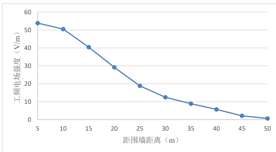
图 5.11-2 围墙外电场强度随距离变化图
